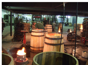
ワイン樽の製造過程 Manufacture process
